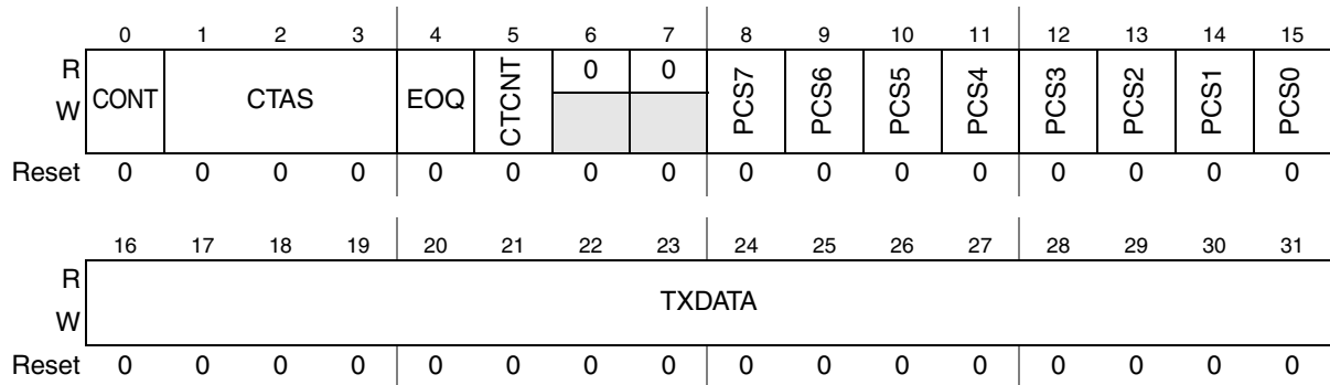
Figure 20-8. DSPI PUSH TX FIFO Register (DSPIx_PUSHR)
