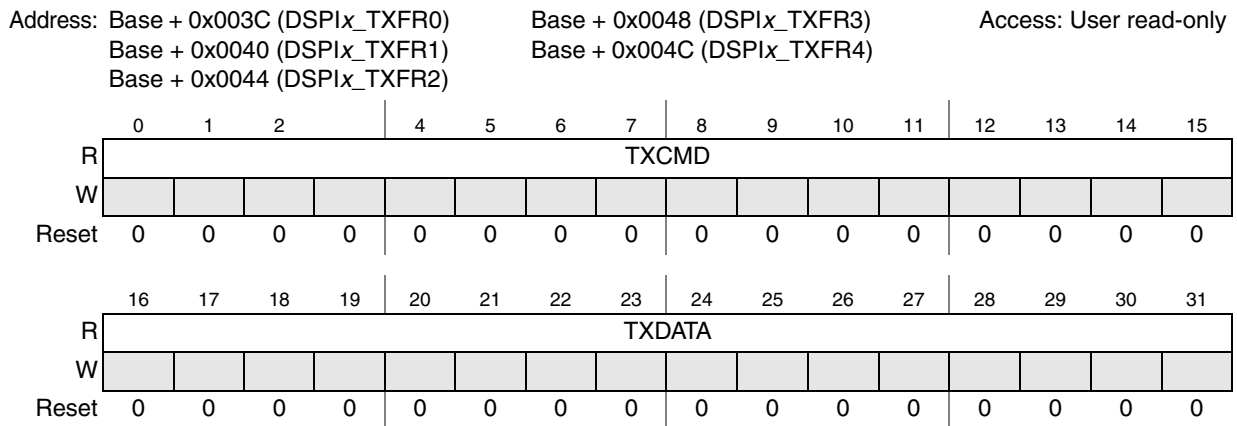
Figure 20-10. DSPI Transmit FIFO Register 0–4 (DSPIx_TXFRn)
