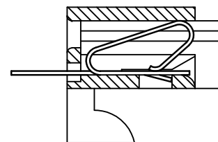
OPTIONAL CORE
