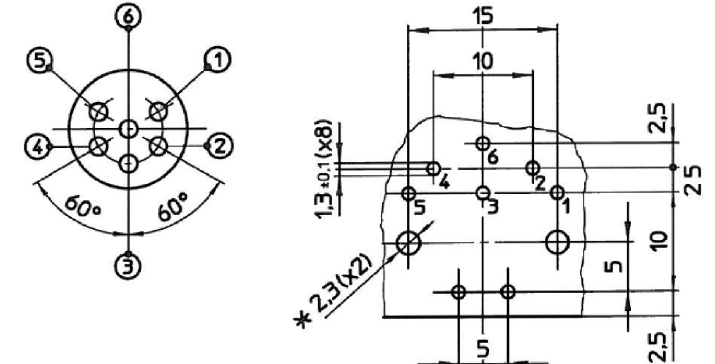
671-0700 Foot Print
