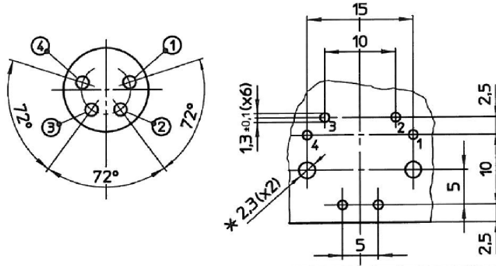
671-0400 Foot Print
