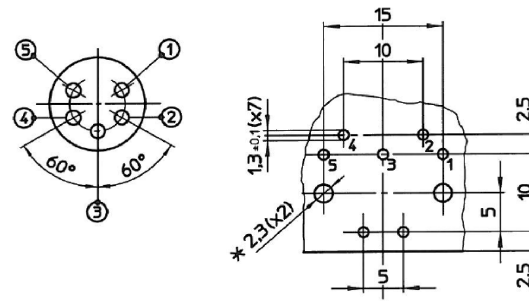
671-0510 Foot Print
