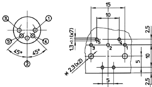
671-0500 Foot Print
