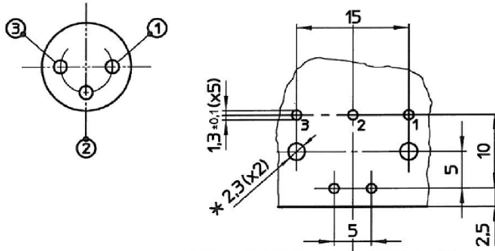
671-0400 Foot Print
