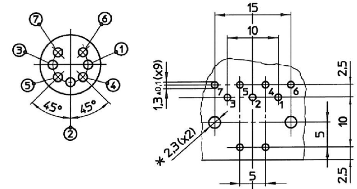
671-0800 Foot Print
