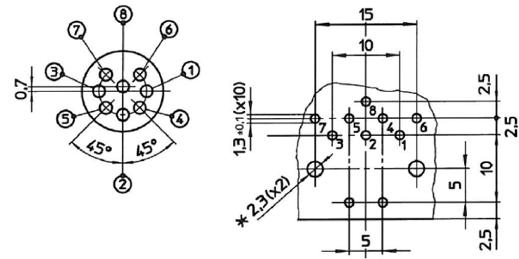
671-0800 Foot Print
