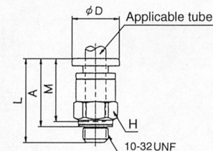
KQ2H05-M5
