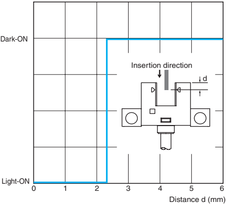
EE-SX910
