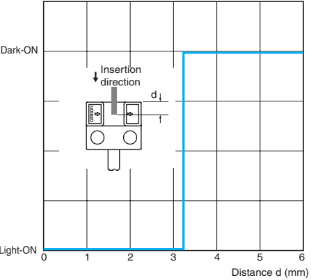
EE-SX911
