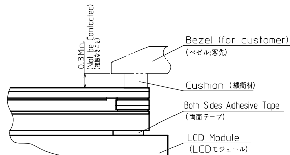
SECTION D-D(NTS)
