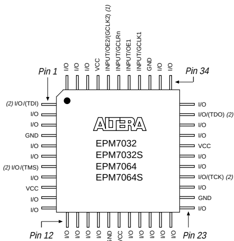
44-Pin TQFP
