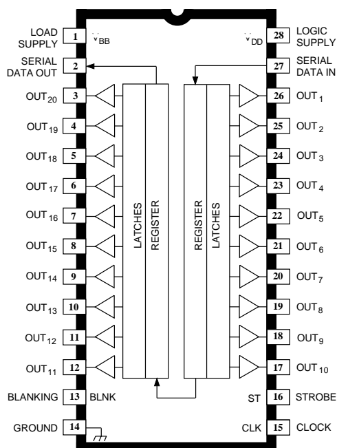
A6812xA (DIP)
