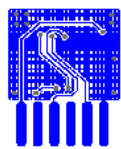
Bottom Layer
