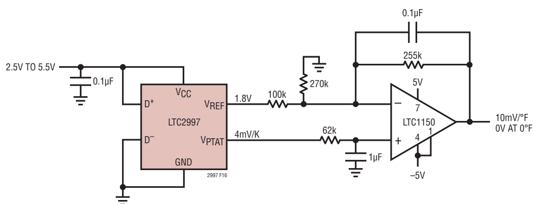
Figure 16. Fahrenheit Thermometer
