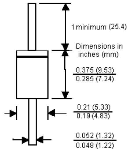
DO-201AD
