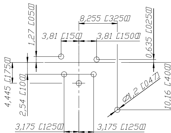
Print-Bohrplan (Bestückungsseite) PCB-Layout (component side)
