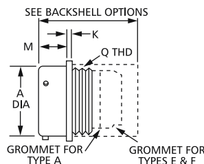
CRIMP KPSE01 (MS3121)
