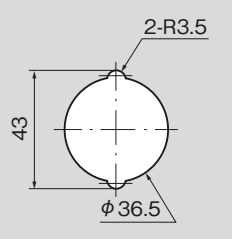
パネル穴明け寸法 Panel drilling dimensions
