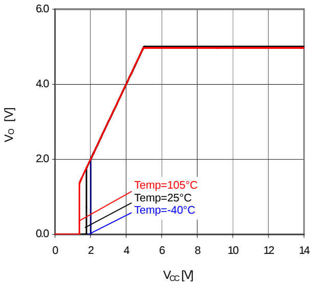
Fig.27 V_{CC}-V_o ( I_o=0\text{mA} )
