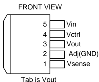
TO263-5L
