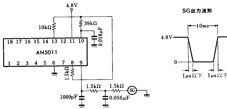
Test Circuit 17 (CHU, CHD 入力による順次選局動作)
