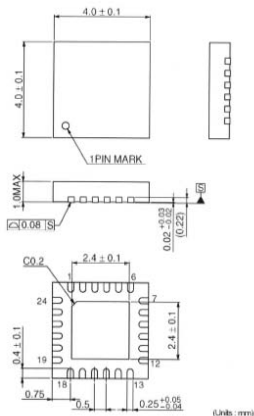
VQFN024V4040VQ
