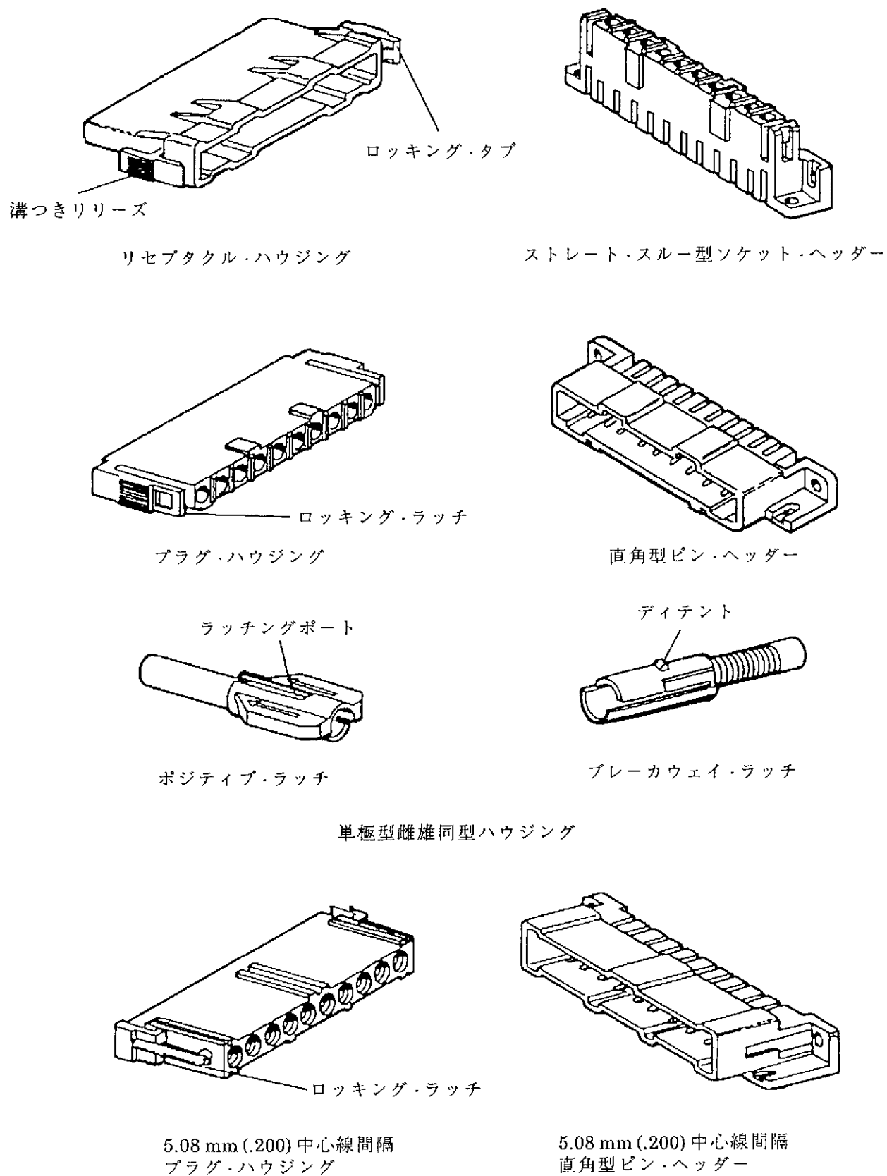
Fig. 1 製品の形状 (終り)
