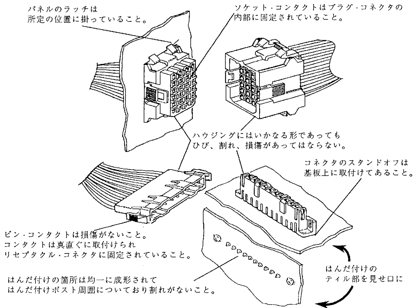
Fig. 10 目視検査用製品図
