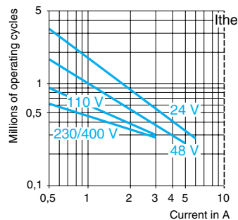
XE2SP21•1, XE2SP2141
