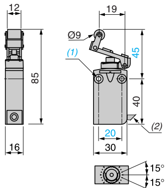
ZCMD21L08*** + ZCE 24
