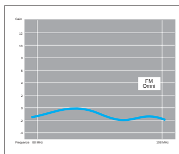
FM Omni-antenn
