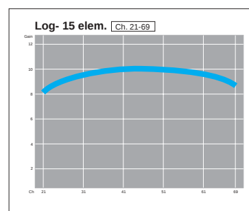
Log-periodisk UHF
