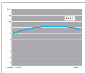
DAB 5
