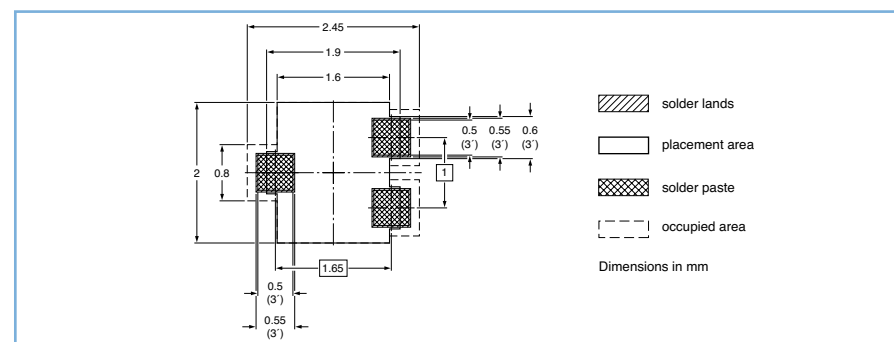
SOT663
