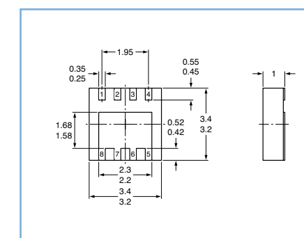
SOT873 (HVSON8)
