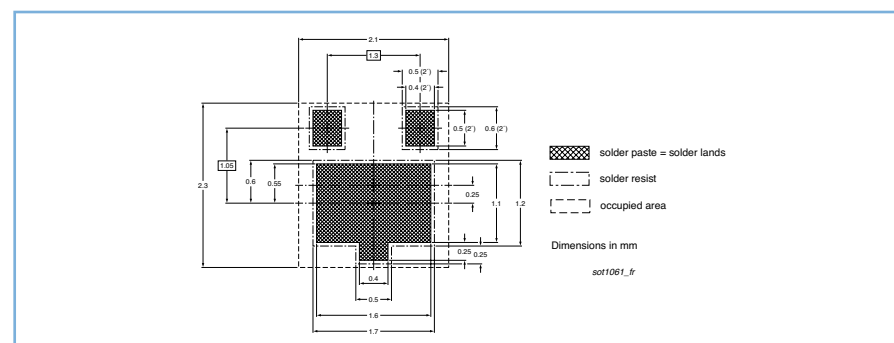
SOT1061
