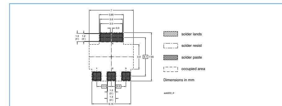
SOT223 (SC-73)
