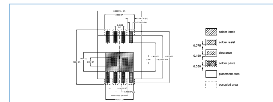
SOT873 (HVSON8)
