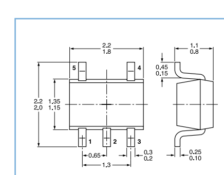
SOT353 (SC-88A)
