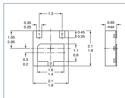
SOT1061
