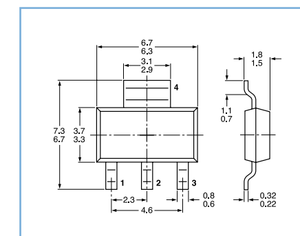
SOT223 (SC-73)
