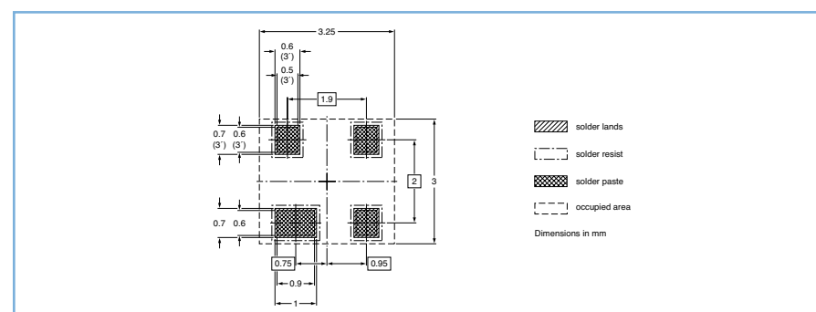
SOT143B
