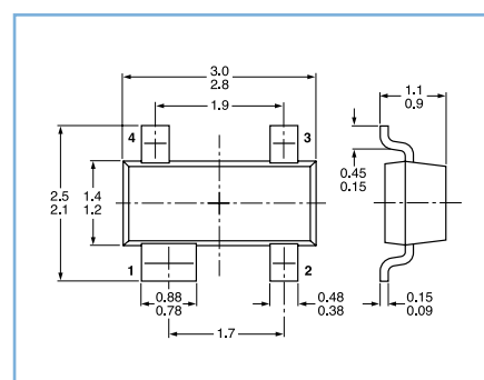
SOT143B
