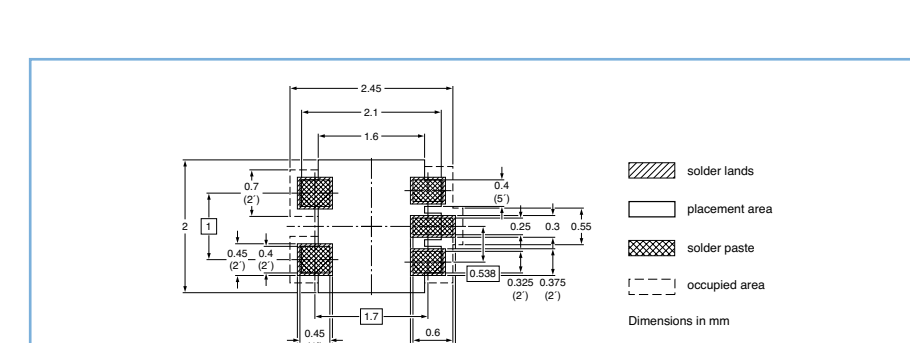
SOT353 (SC-88A)
