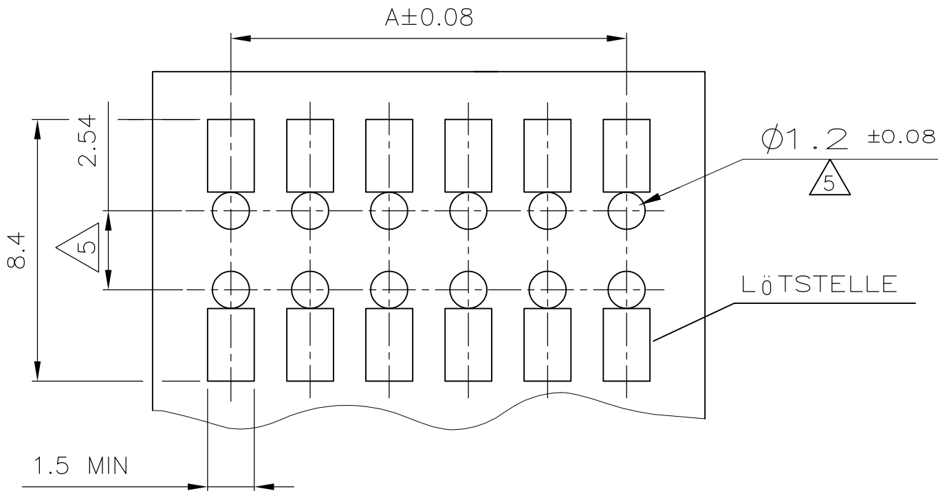
EMPFOHLENES LEITERPLATTEN LAYOUT
