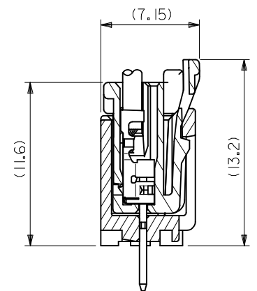
嵌合断面図
