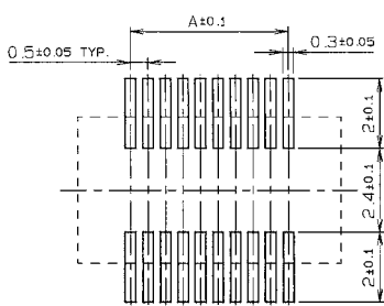
基板取付け寸法 MOUNTING LAYOUT
