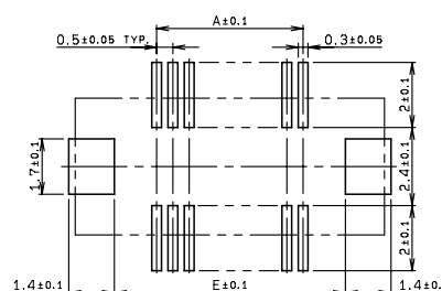
基板取付け寸法 MOUNTING LAYOUT
