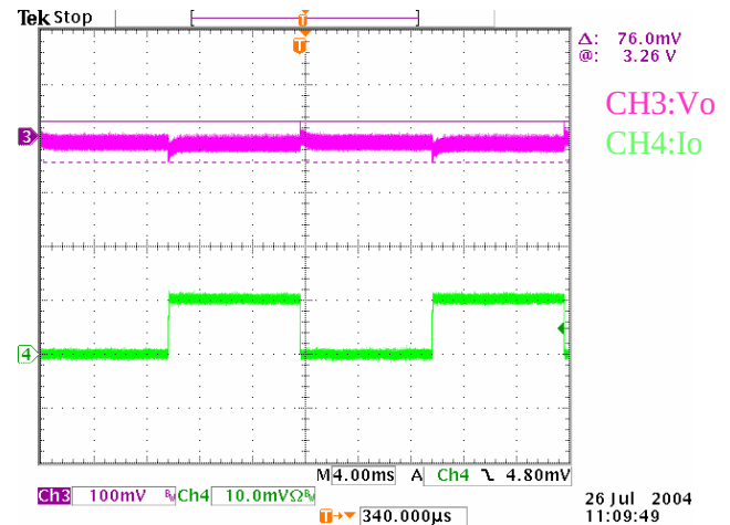
Transient response(0-5A).
