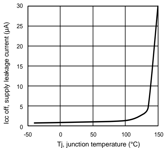
Figure 4 – Icc off (μA) VsTj (°C)
