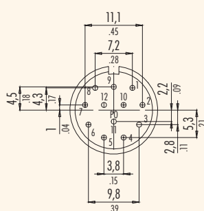
Stiftkontakteinsatz male insert
