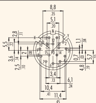
Stiftkontakteinsatz male insert
