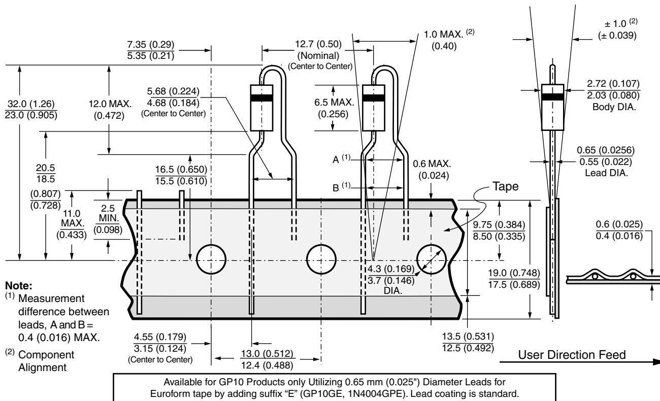
Fig. 3 - Euroform
