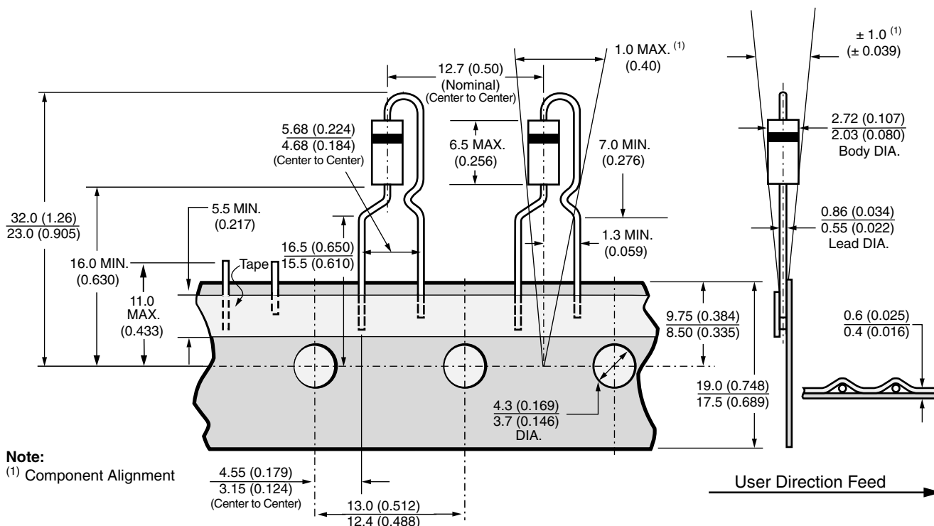
Fig. 4 - Panasert
