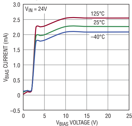
V_{BIAS} Quiescent Current
