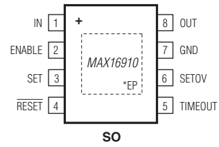
SO
