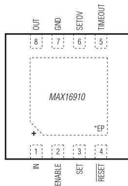
TDFN
