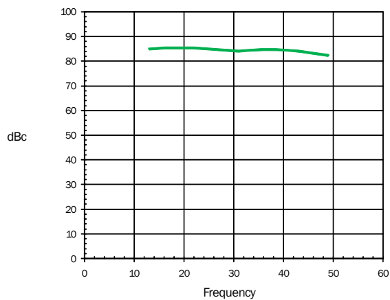
\text{CSO } V_{DD}=12\text{V}
