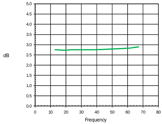
\text{CTB } V_{DD}=12\text{V}
