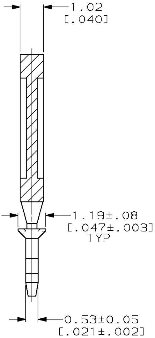
SECTION A-A
