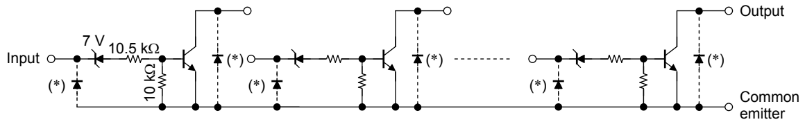
TD62502FNG
