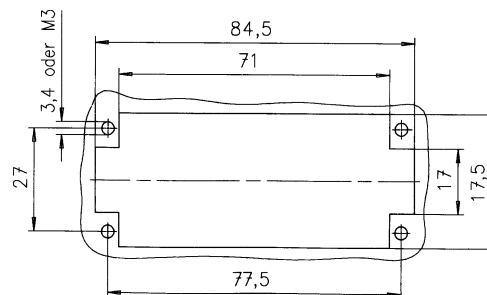
Montageausschnitt (Kontaktträger) Panel cut out (insert)
