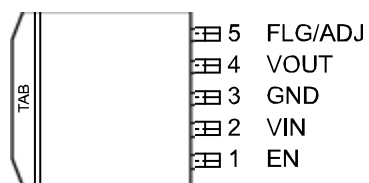
S-PAK-5 (R)
