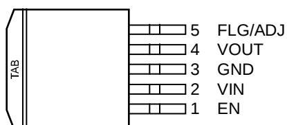
TO-263-5 (U)
