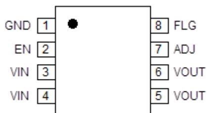
3mm × 3mm DFN (ML)
