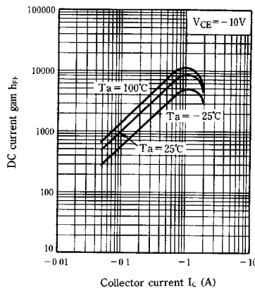
h_{FE} - I_C
