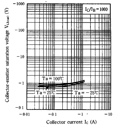
V_{CE(sat)} - I_C
