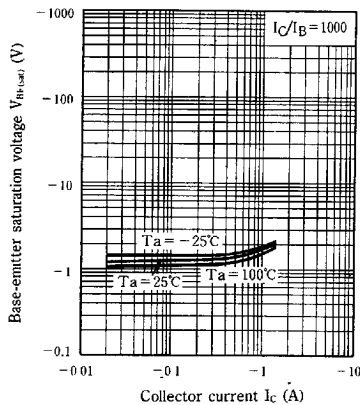
V_{BE(sat)} - I_C
