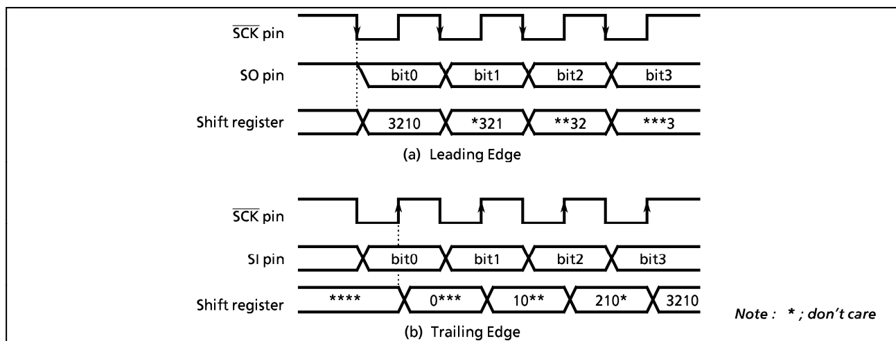
Figure 2-39. Shift Edge
