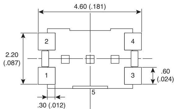
P.C.B. Layout
