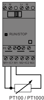
3Leitertechnik
