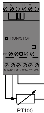
3Leitertechnik
