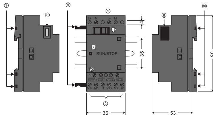
LOGO! AM2 AQ (0 ... 10 V DC oder 0/4 ... 20 mA)
