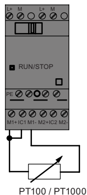
2Leitertechnik
