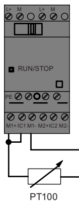
2Leitertechnik
