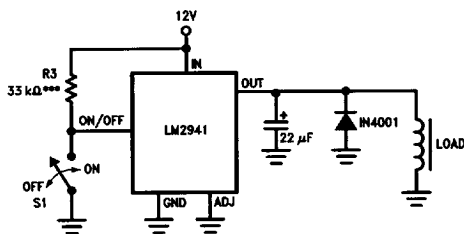
1A Switch
