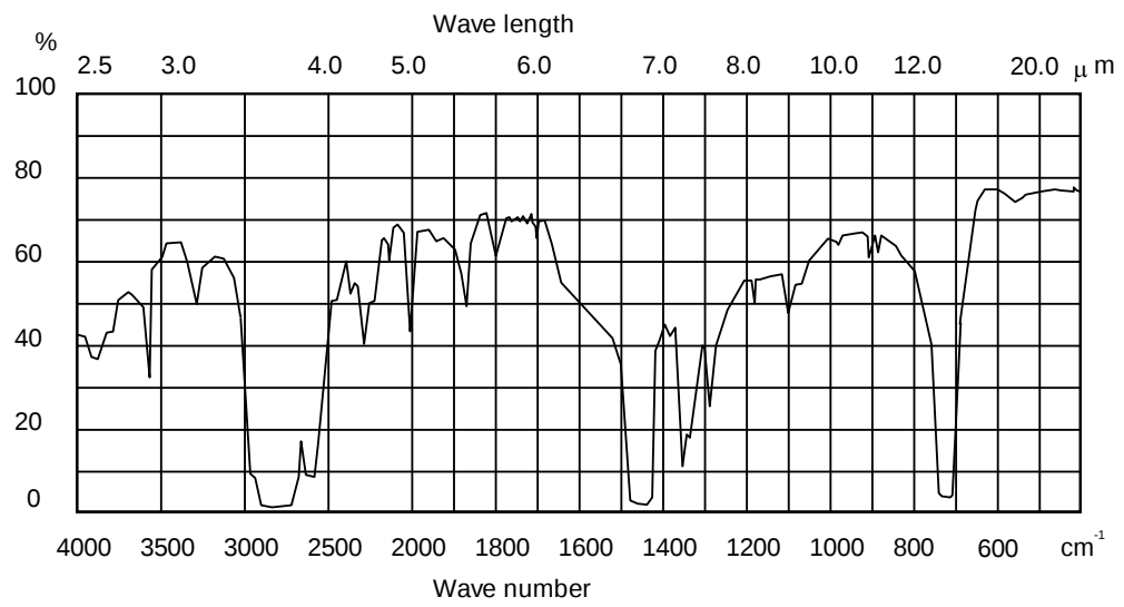
第 2 図 赤外分光透過特性
