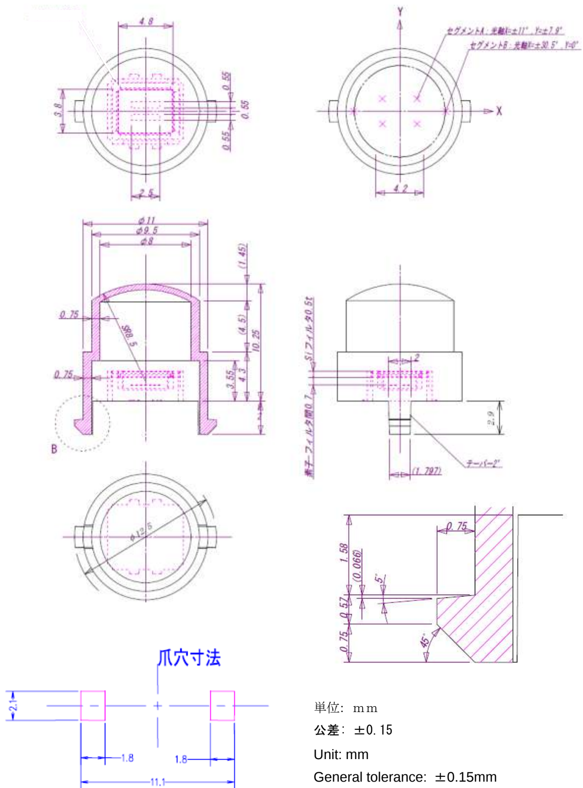
第 1 図 外形寸法図
