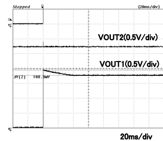
VIN=5.5V,EN2=H(ON)
