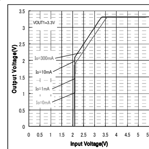
Fig.6. Output Voltage (VOUT1=3.3V)
