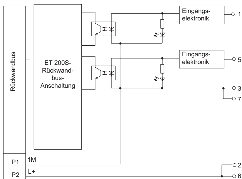
Bild 1-1 Prinzipschaltbild des 2DI DC24V ST
