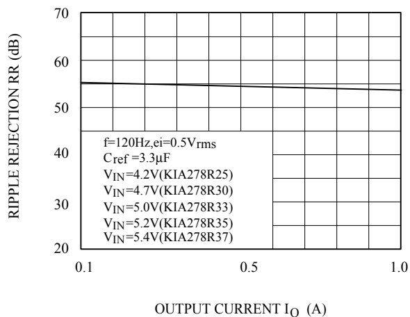
Fig.10-2 I_O - RR
