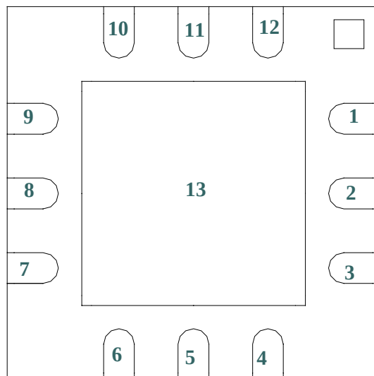
Bottom Side
