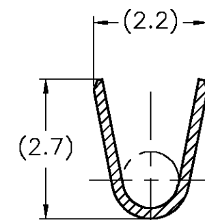
断面 C-C SECT.
