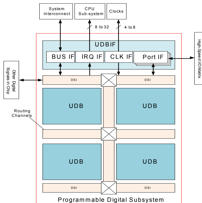
Figure 4. UDB Array
