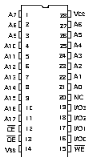
SOJ
