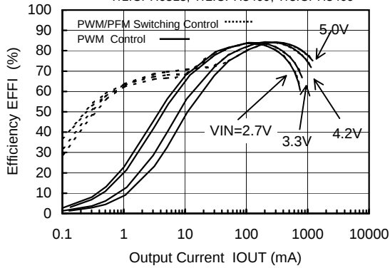
FOSC=300kHz, VOUT=3.3V
