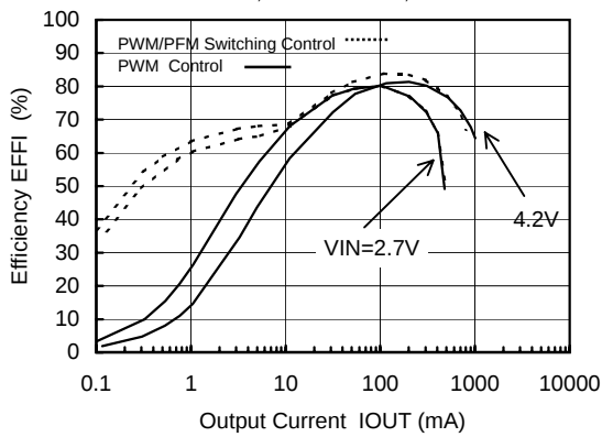
FOSC=300kHz, VOUT=3.3V
